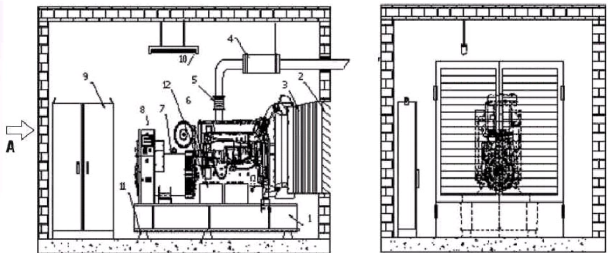
ВИД А
