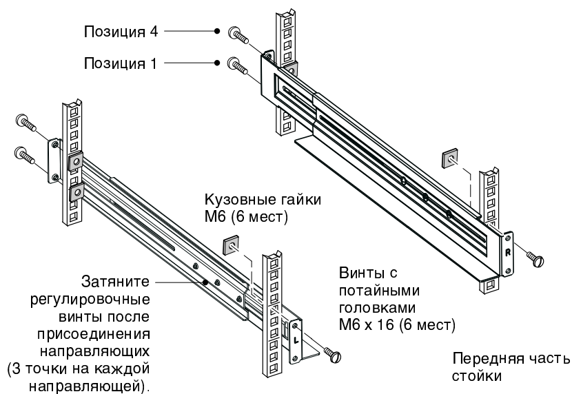
Рисунок 5. Крепление направляющих
