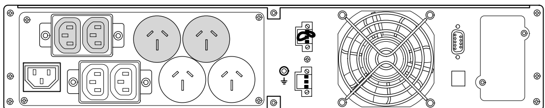
Рисунок 38. Модель PW9130G2000R-XL2UAU
