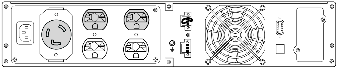
Рисунок 36. Модель PW9130G2000R-XL2U
