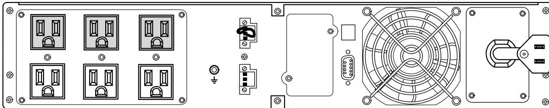
Рисунок 33. Модель PW9130L1500R-XL2U
