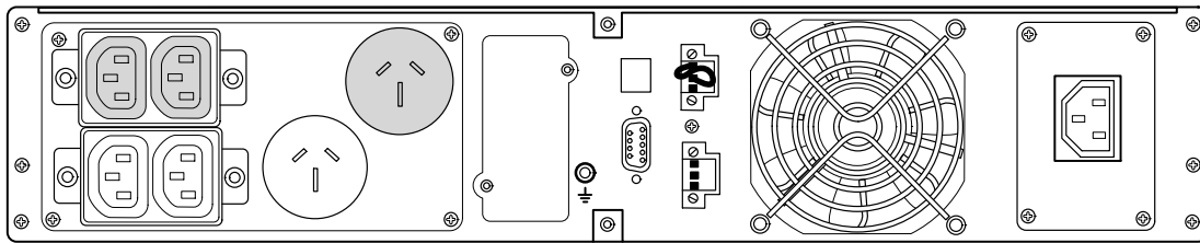
Рисунок 31. Модель PW9130G1000R-XL2UAU
