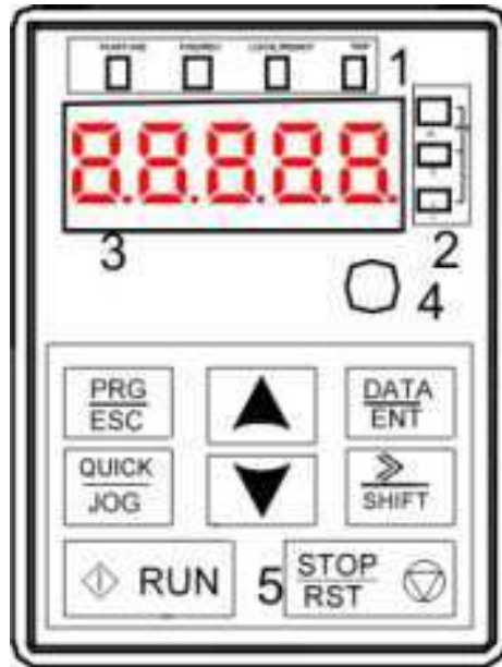
Рис. 6-1 Панель управления
