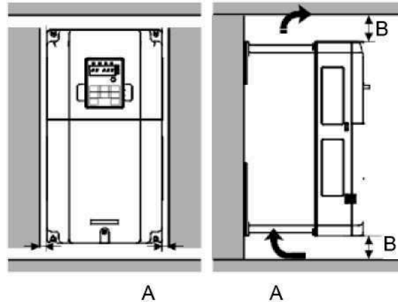
Рисунок 4-2. Вентиляционные промежутки
