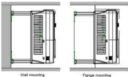
Рис. 3-1 Установка ПЧ
