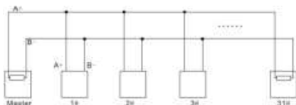
Рис. 3 Подключение «Шина»
