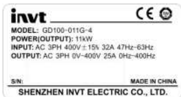
Рис. 2-1 Шильдик ПЧ
