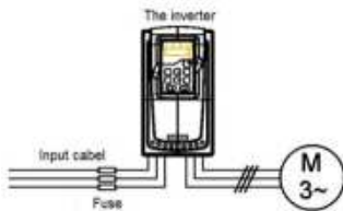
Рис. 3-10 Подключение предохранителей
