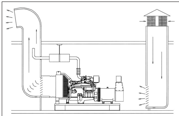
Figure 5.4. Воздушная вентиляция
