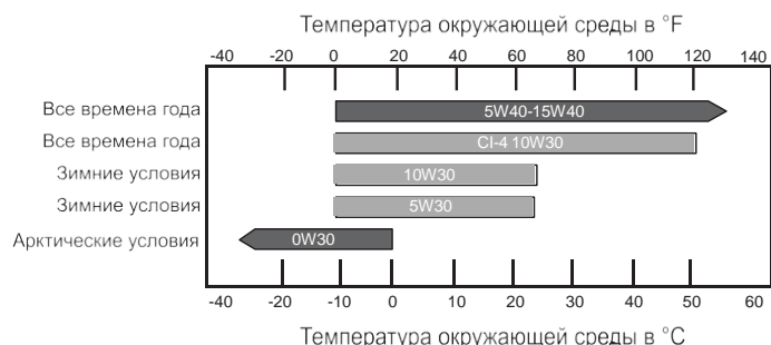
Рис. 9.1. Рекомендуемая вязкость/сорт масла по SAE в зависимости от температур окружающей среды
