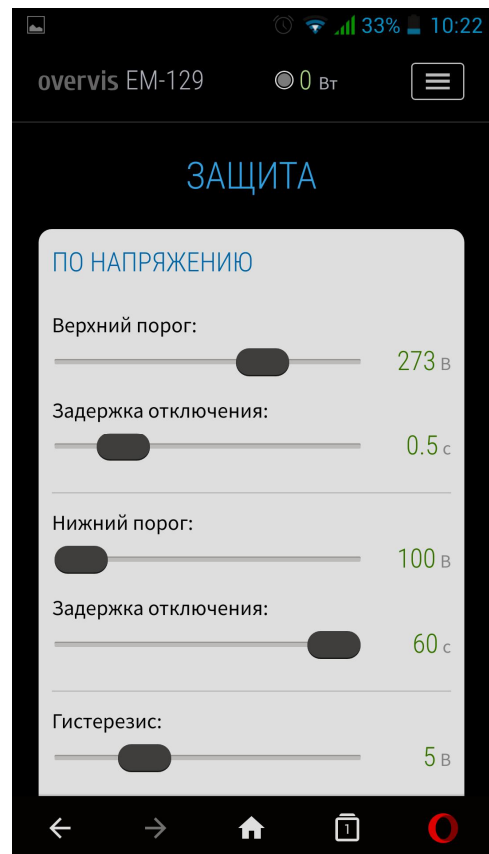
Рисунок А5 – Защита по напряжению
