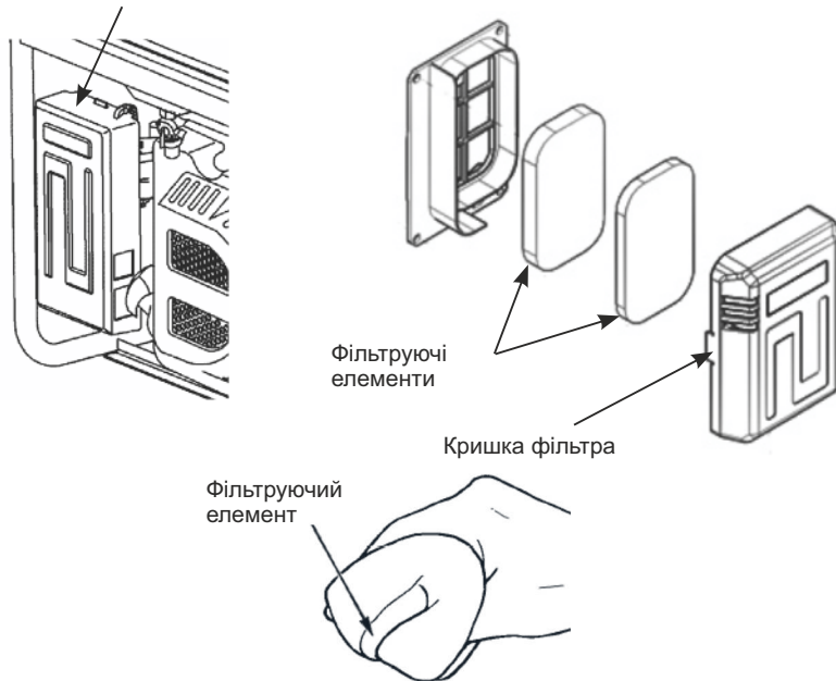
Повітряний фільтр
