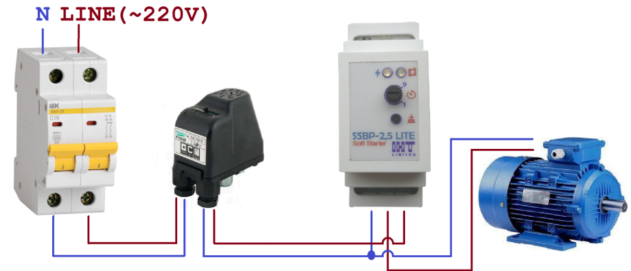
мал. 4 Можлива схема підключення при автоматичному режимі
