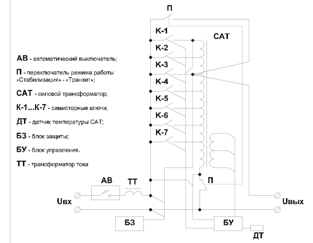
Рис. 3. Структурная схема блока фазной стабилизации
