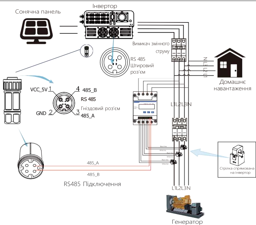
Малюнок 7.16 Схема підключення лічильника CHNT
