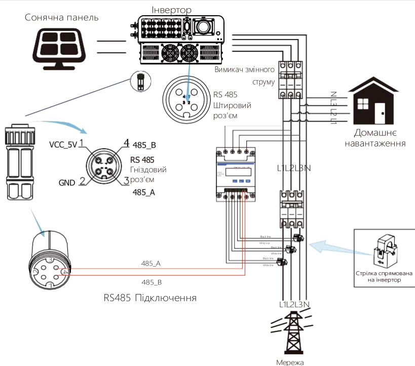
Малюнок 7.14 Схема підключення лічильника CHNT
