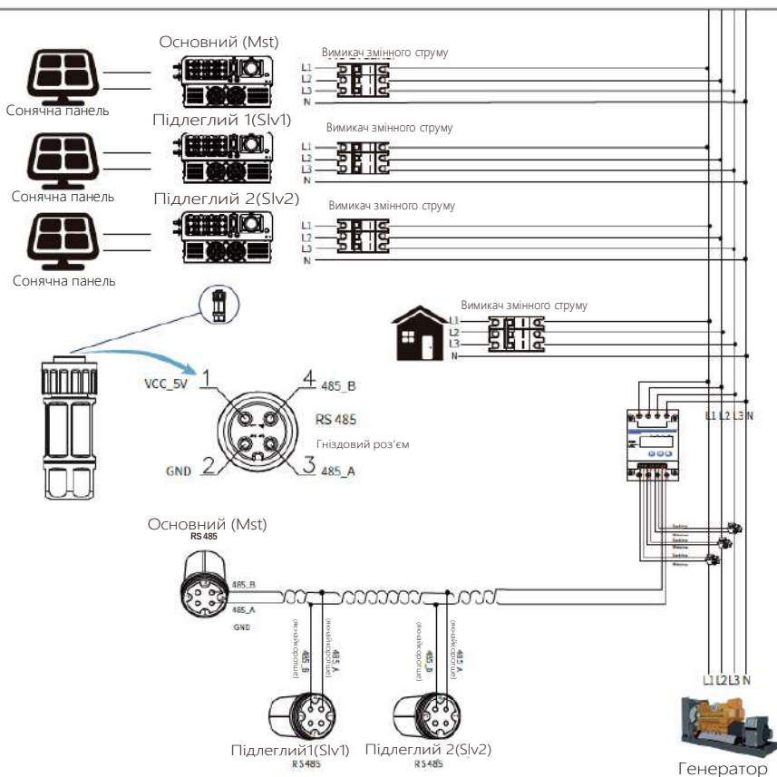
Малюнок 7.33 Схема підключення СНТ (Прохідна схема)
