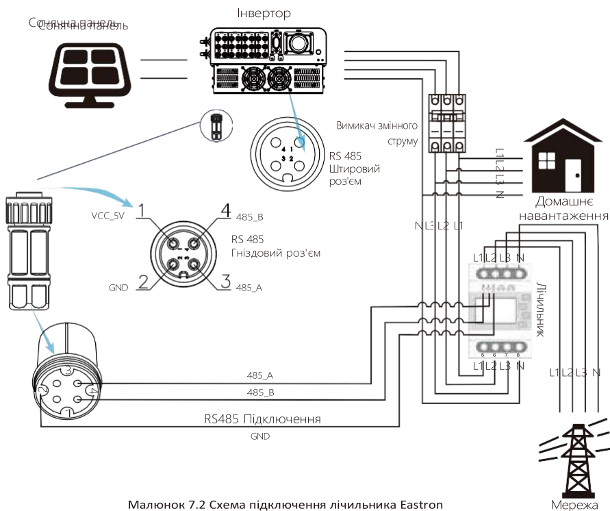
Малюнок 7.2 Схема підключення лічильника Eastron
