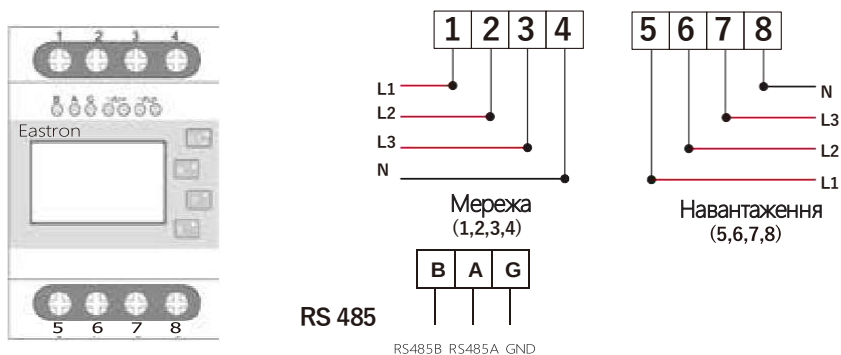
Малюнок 7.3 Лічильник Eastron
