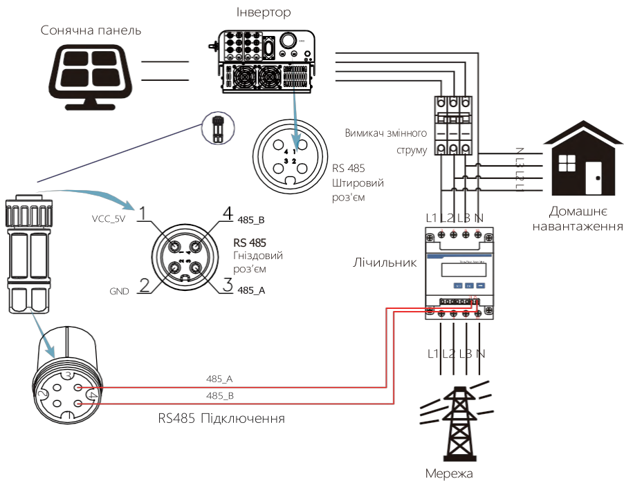
Малюнок 7.10 Схема підключення лічильника CHNT meter
