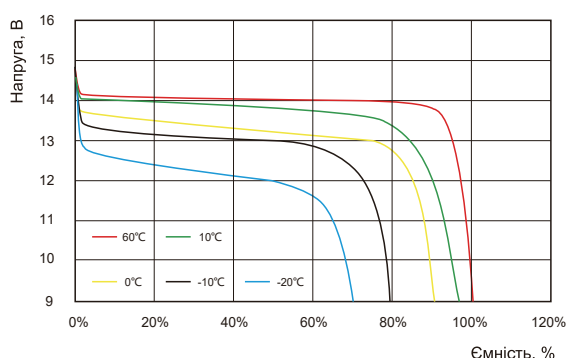
Криві розряду при різних температурах
