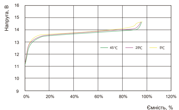
Криві заряду при різних температурах
