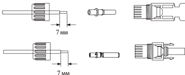
Малюнок 5.3 Розбирання накидної гайки роз'єму
