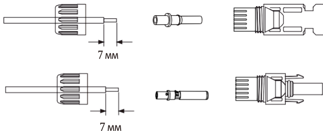
Малюнок 3.3 Розбирання накидної гайки роз'єму
