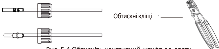
Рис. 5.4 Обтисніть контактний штифт до дроту
