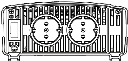
Рисунок 3. Розташування розеток на корпусі стабилизатора КилоГерц 1-8
