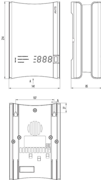
Рисунок 4. Габаритні та установочні розміри стабілізатору КилоГерц У 1-3 та 1-5
