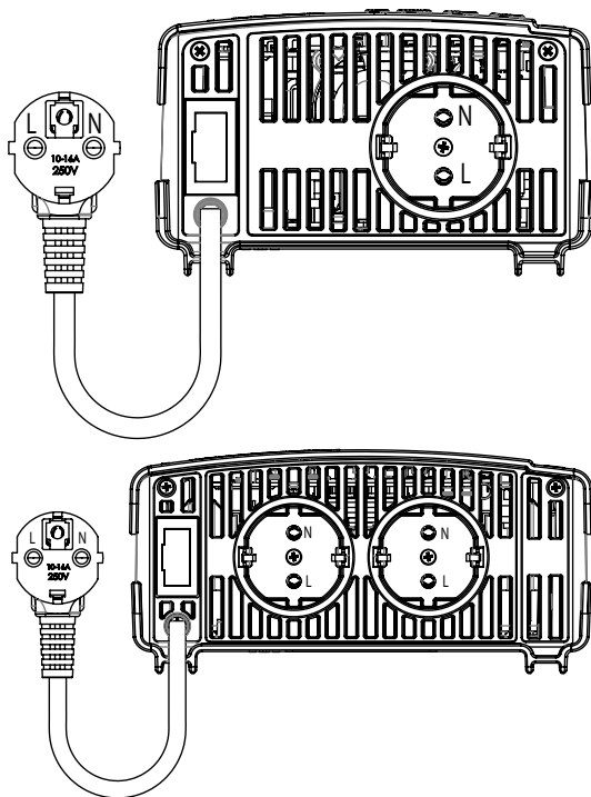
Малюнок 7. Розташування контактів «Фаза» та «Нуль» на вилці та розетці КілоГерц
