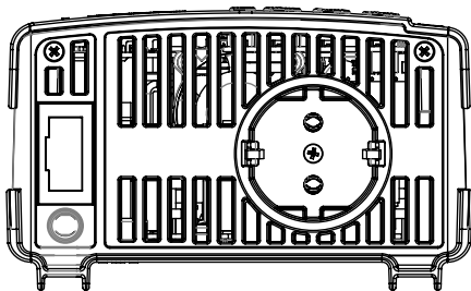
Рисунок 2. Розташування розеток на корпусі стабилизатора КилоГерц 1-3 и 1-5
