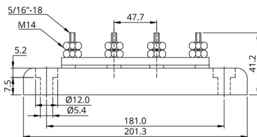
Шина 250 А з 4 гвинтовими клеммами та кришкою
